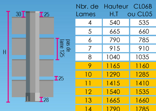
Assemblage Ranch tablier ajouré PB09 (100)
