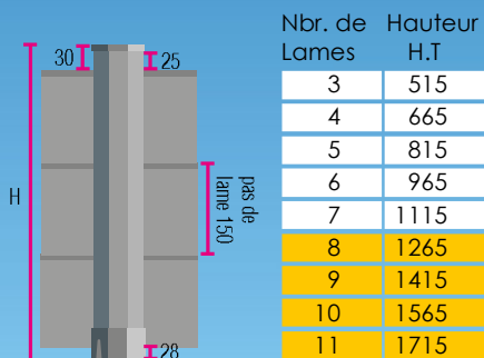
Assemblage Ranch tablier plein PB06 (150)
