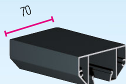
Support de fixation pour pilier CL09
