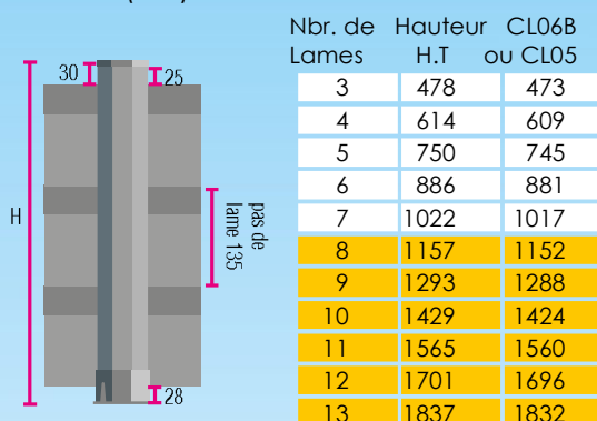
Assemblage Brise vue CL07 (136)
