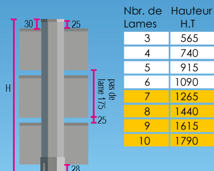
Assemblage Ranch tablier ajouré PB06 (150)
