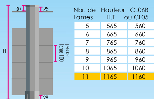
Assemblage Ranch tablier plein PB09 (100)
