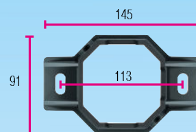
ST36 (pied) support de fixation pour poteau de clôture
