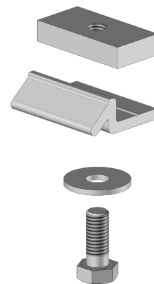
PV0405 : Nb = Nb panneau x 4
