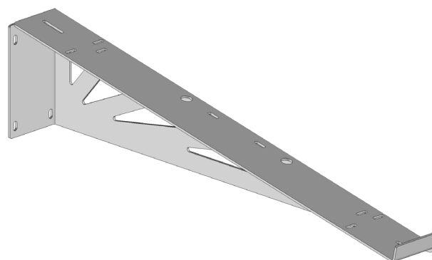
EQPV08-1 ou EQPV09-1 Droite Nb = 1 par panneau PV EQPV08-1 Compatible panneaux 1100mm à 1150mm EQPV09-1 Compatible panneaux 1020mm à 1070mm
