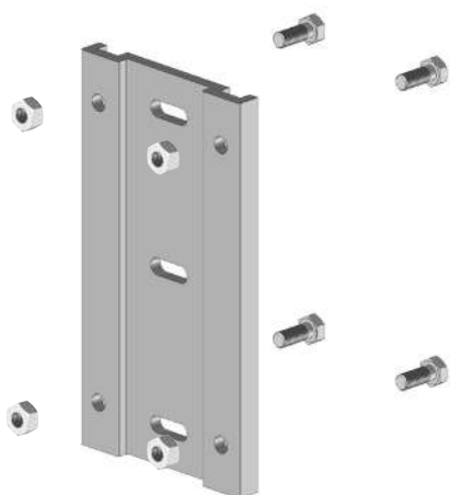
PS135M250 + DIN933M10x25mm + DIN934M10 : Nb = Nb équerre
