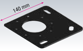
Suporte de fixação ao solo: ST38
