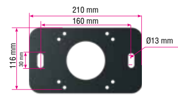
Suporte de fixação ao solo : ST45
