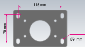
Suporte de fixação ao solo: ST55
