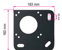
Suporte de fixação ao solo : ST4502
