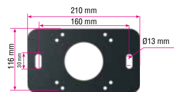
Suporte de fixação ao solo : ST45
