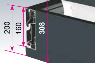
Largura de lâmina a lâmina 175mm Lâmina : PBS043
