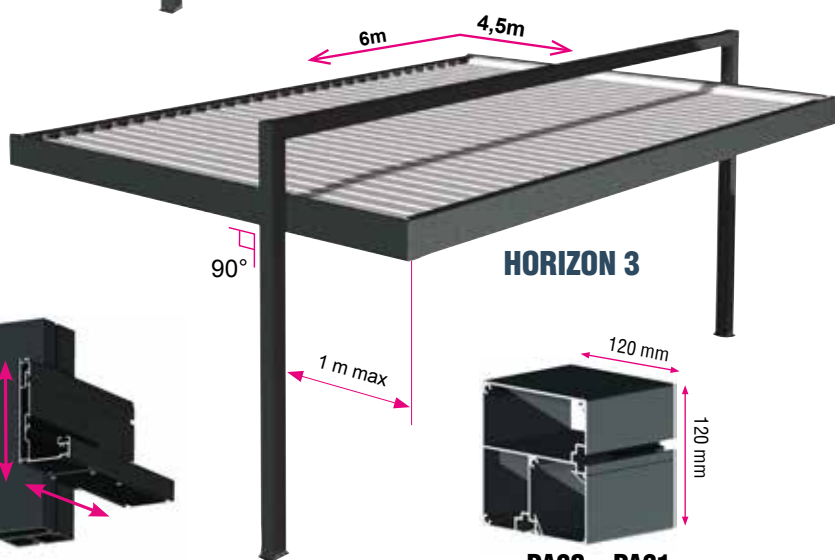
PA30 + PA31 Postes da versão com arco
