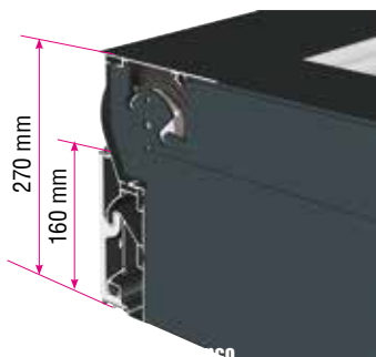
Espaço das lâminas recolhidas 20% do avanço
