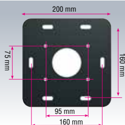
Suporte de fixação ao solo : ST4510
