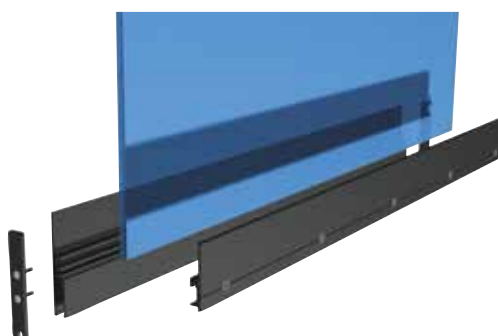
Perfil inferior, base deslizante
