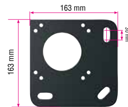
Suporte de fixação ao solo : ST4502
