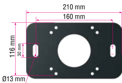
Suporte de fixação ao solo : ST45
