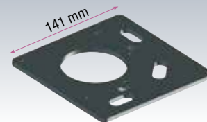
Suporte de fixação ao solo : ST48
