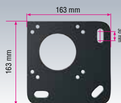
Suporte de fixação ao solo : ST4502
