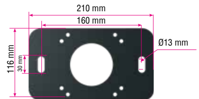
Suporte de fixação ao solo : ST45
