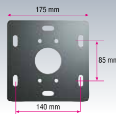
Suporte de fixação ao solo: ST4509
