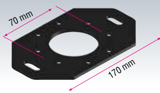
Suporte de fixação ao solo: ST3802
