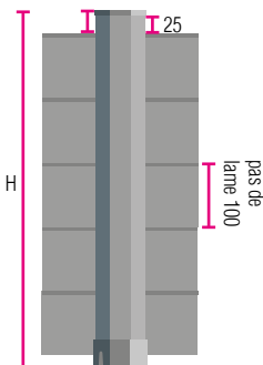
Assemblage Ranch tablier plein PB09 (100)
