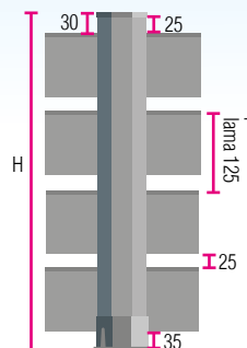
Paneles espaciados Ranch PB09 (100)
