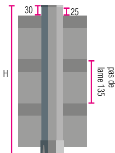
Assemblage Brise vue CL07 (136)
