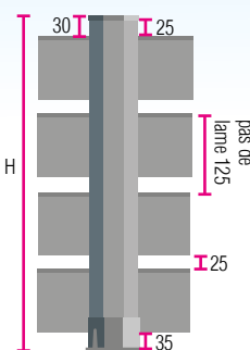
Assemblage Ranch tablier ajouré PB09 (100)
