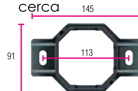
ST3603A (pie) soporte de fijación para poste de cerca
